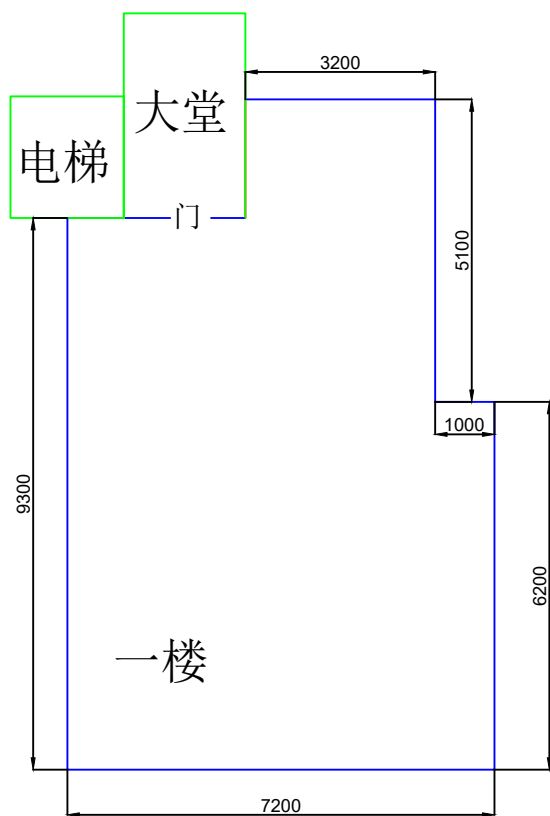
嘉善亭溪苑21-1-101尺寸图
